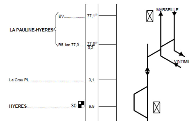
Figure 2.4 – Antenne d'Hyères
