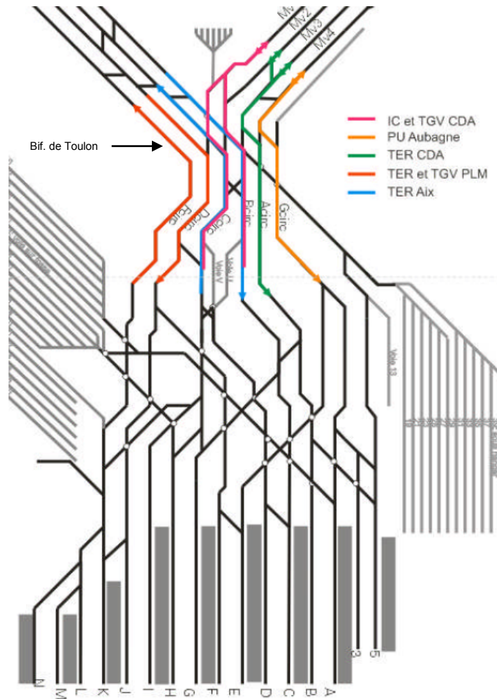
Figure 4 : les tubes de circulation au niveau de la zone d'échanges
