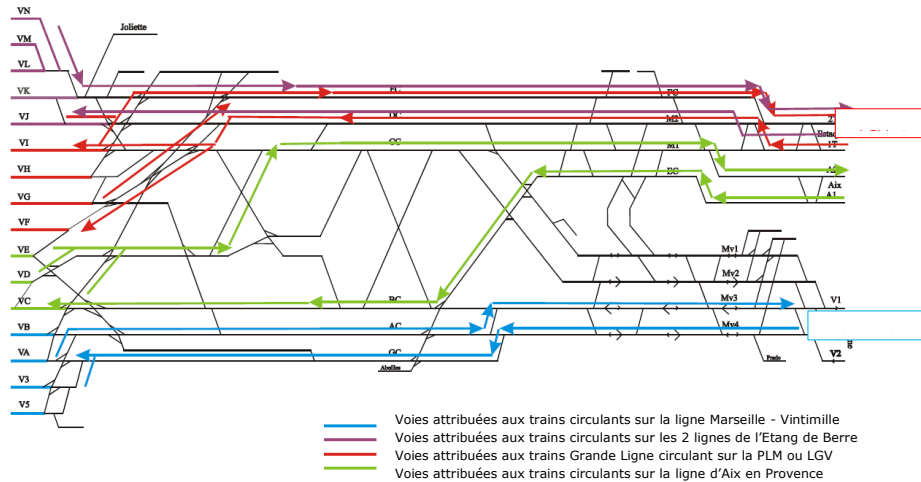
Exploitation par tube permettant de réduire les conflits et les cisaillements
